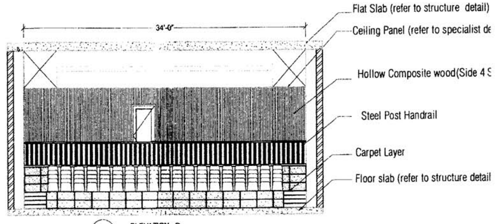
A-415 ELEVATION - D SCALE: 1/8" = 1'-0"
