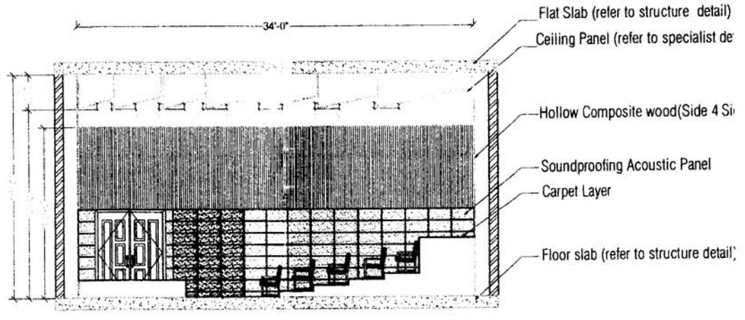
A-415 ELEVATION - C SCALE: 1/8" = 1'-0"
