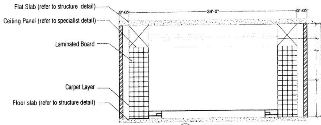
A-415 ELEVATION - B SCALE: 1/8" = 1'-0"
