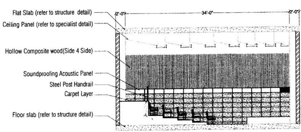
A-415 ELEVATION - A SCALE: 1/8" = 1'-0"
